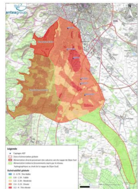
Figure 2 : Carte de vulnérabilité de la zone d'alimentation globale
